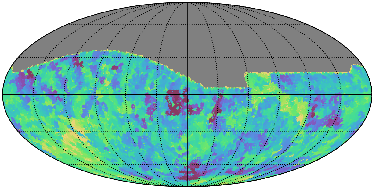
weather_cloudso8v3.4_10yrs All sky i band: Min saturation_mag
