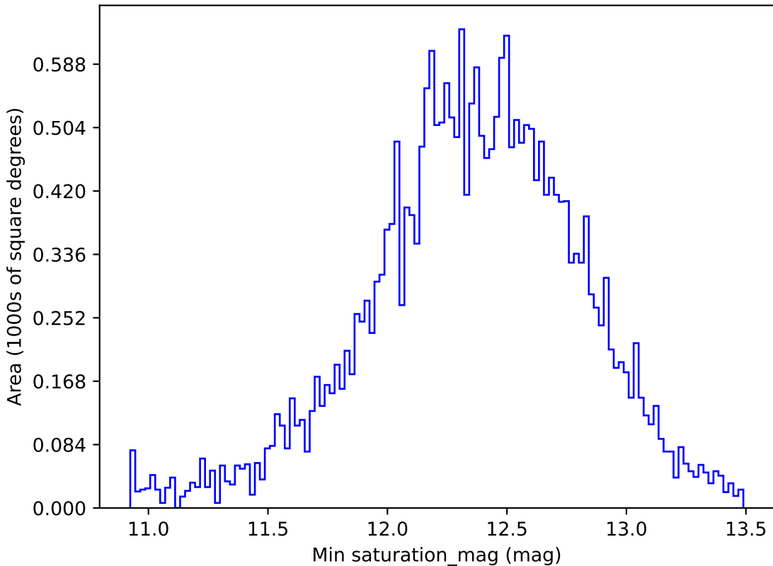
weather_cloudso8v3.4_10yrs All sky i band: Min saturation_mag
