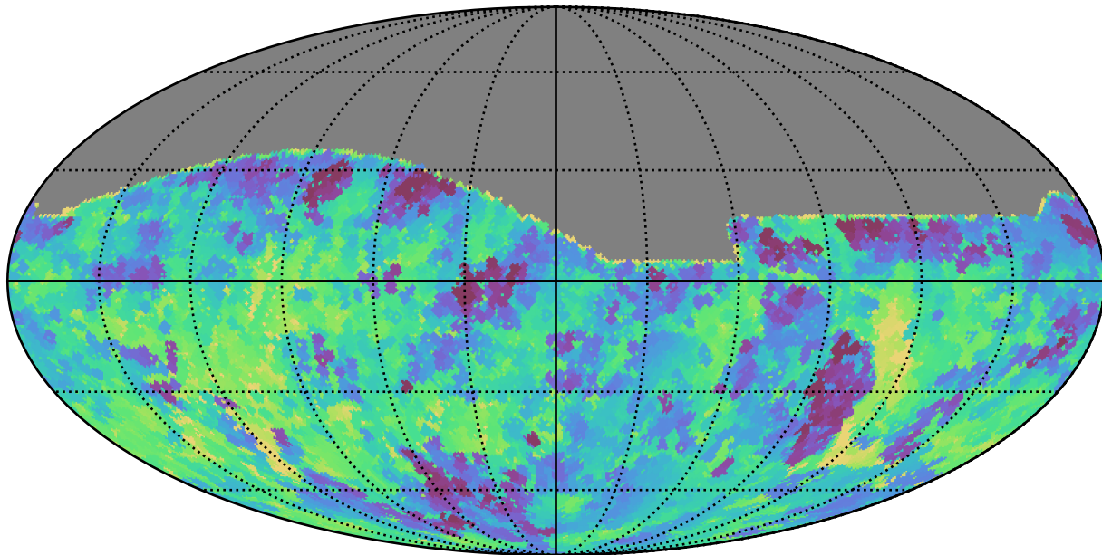
weather_cloudso8v3.4_10yrs All sky g band: Min saturation_mag
