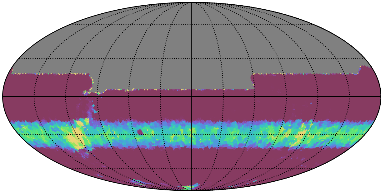
weather_cloudso8v3.4_10yrs All sky y band: Min normairmass
