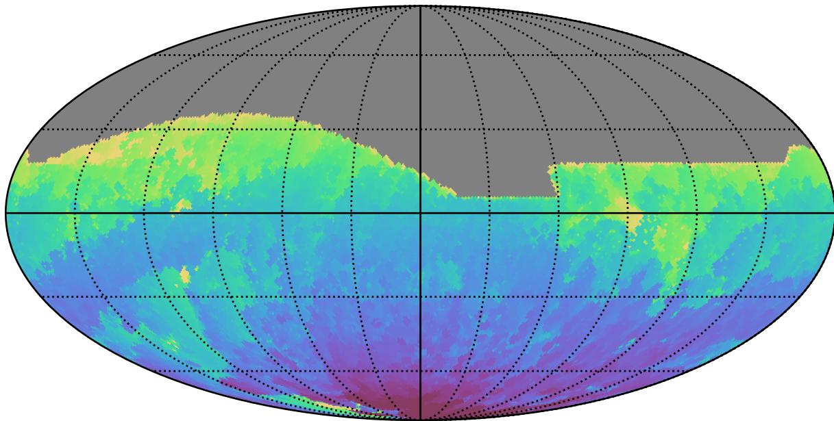
weather_cloudso8v3.4_10yrs All sky z band: Min HA
