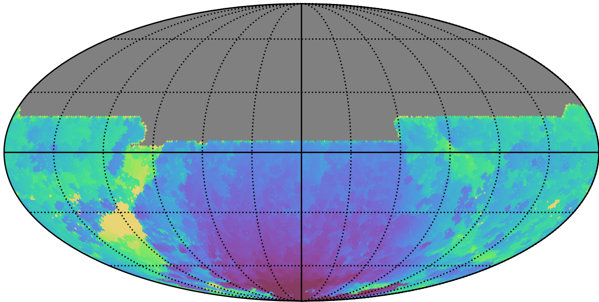
weather_cloudso8v3.4_10yrs All sky y band: Min HA
