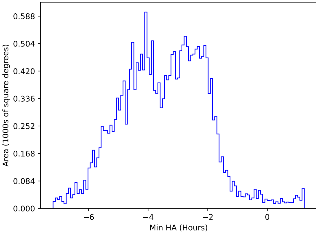
weather_cloudso8v3.4_10yrs All sky y band: Min HA
