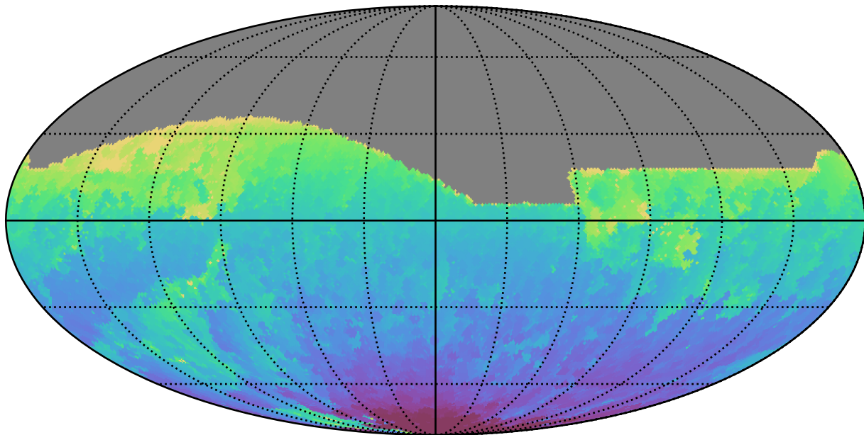
weather_cloudso8v3.4_10yrs All sky i band: Min HA
