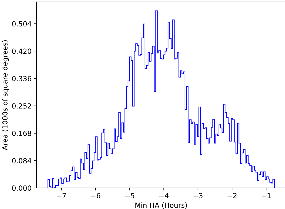
weather_cloudso8v3.4_10yrs All sky g band: Min HA
