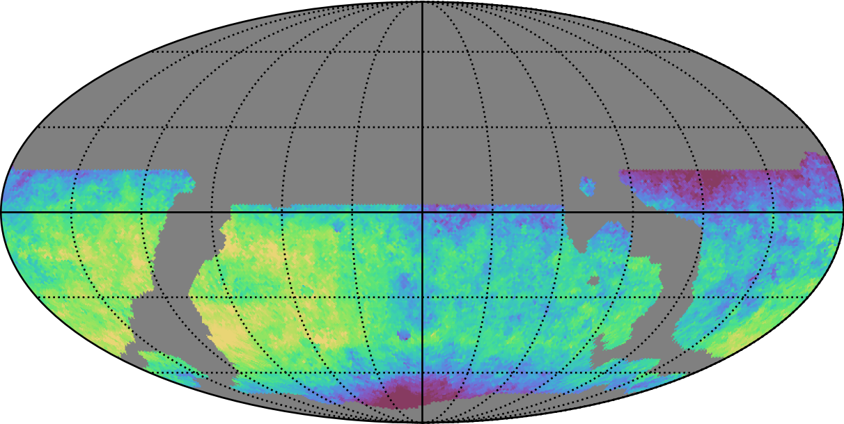
weather_cloudso8v3.4_10yrs WFD y band: Median saturation_mag
