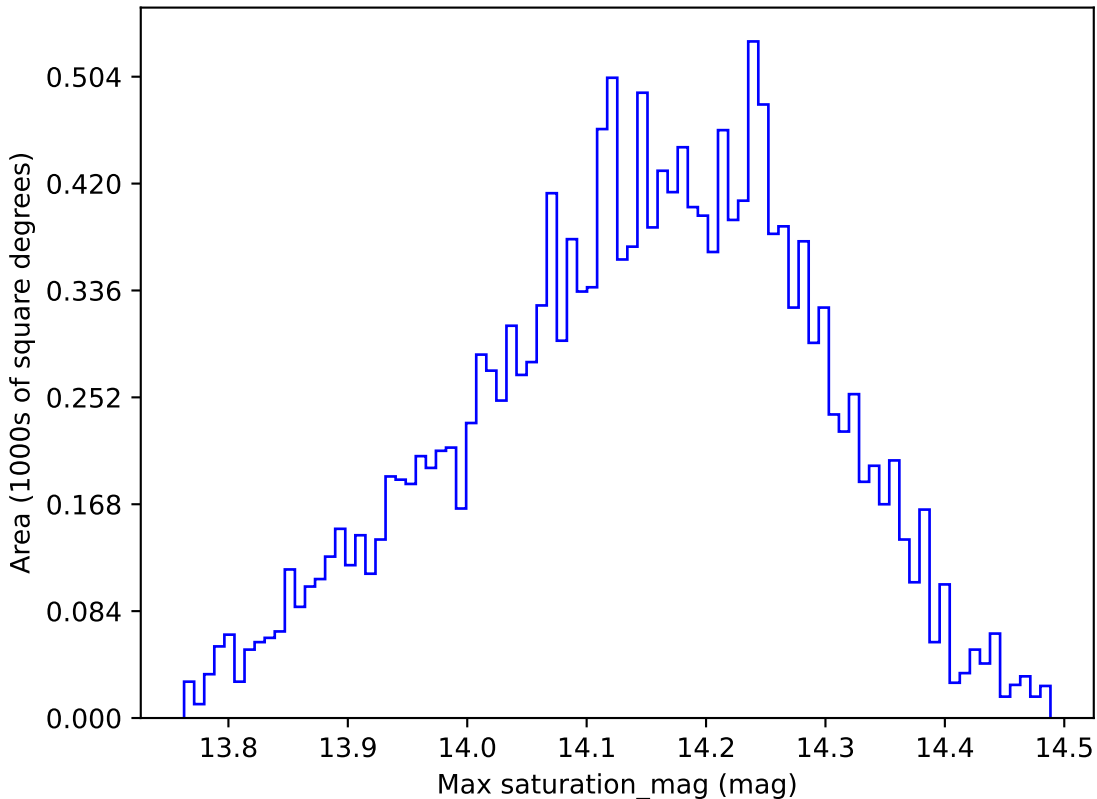
weather_cloudso8v3.4_10yrs WFD y band: Max saturation_mag
