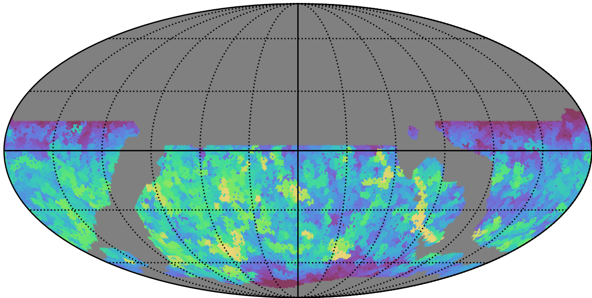
weather_cloudso8v3.4_10yrs WFD i band: Max saturation_mag
