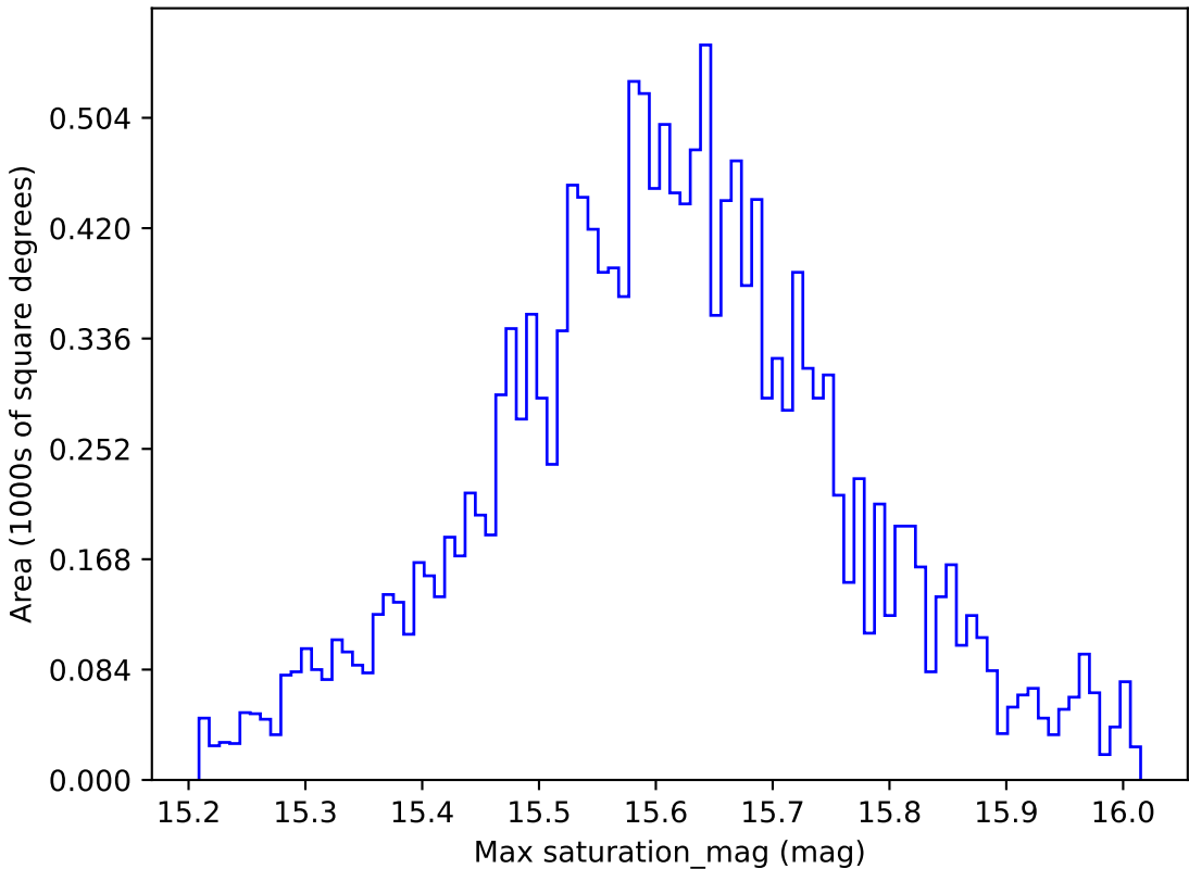
weather_cloudso8v3.4_10yrs WFD i band: Max saturation_mag
