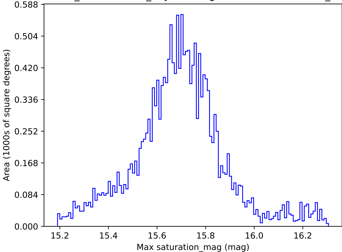
weather_cloudso8v3.4_10yrs WFD g band: Max saturation_mag
