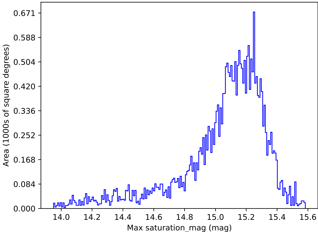
weather_cloudso8v3.4_10yrs All sky z band: Max saturation_mag
