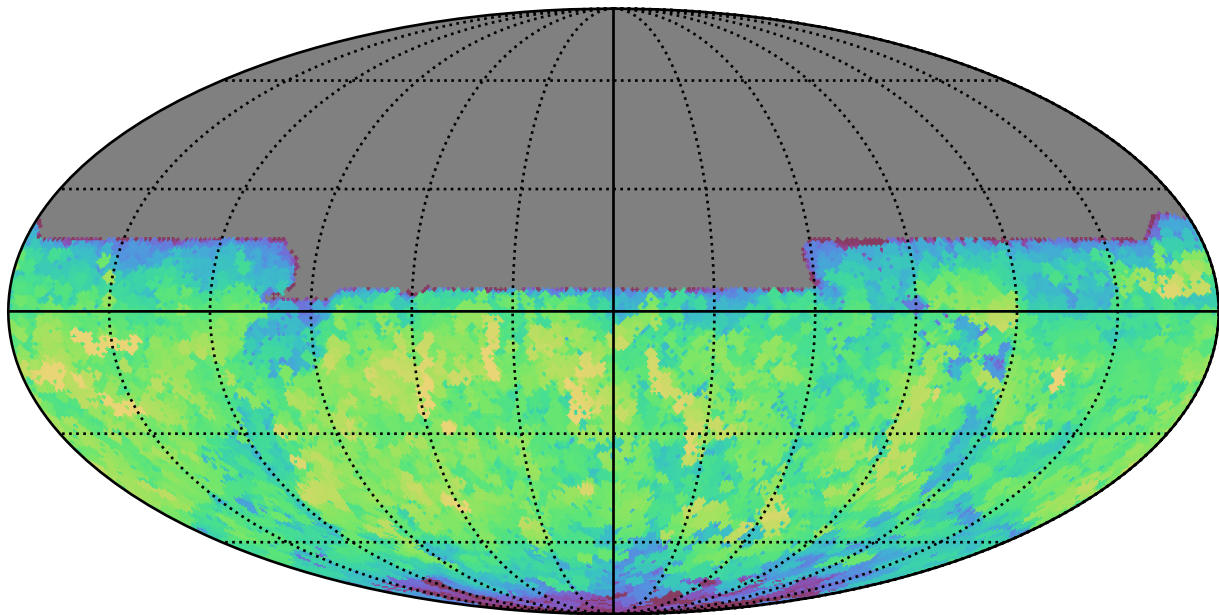
weather_cloudso8v3.4_10yrs All sky y band: Max saturation_mag
