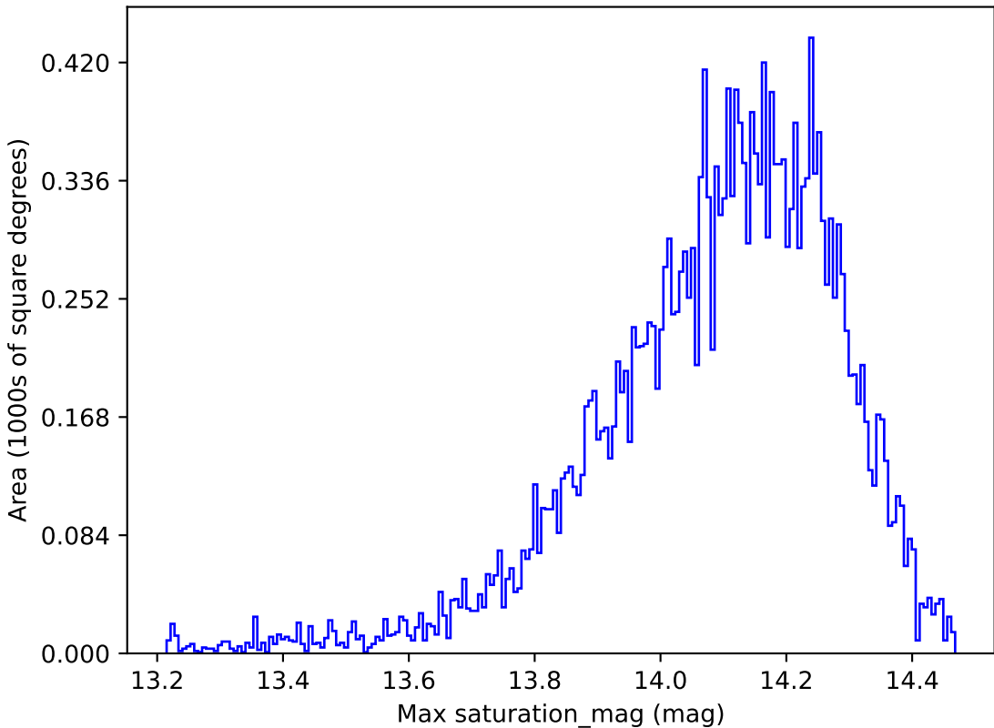
weather_cloudso8v3.4_10yrs All sky y band: Max saturation_mag
