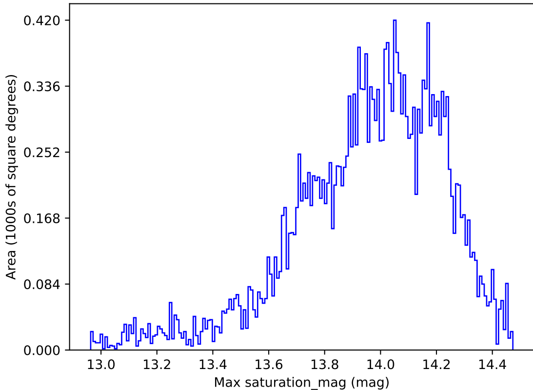
weather_cloudso8v3.4_10yrs All sky u band: Max saturation_mag
