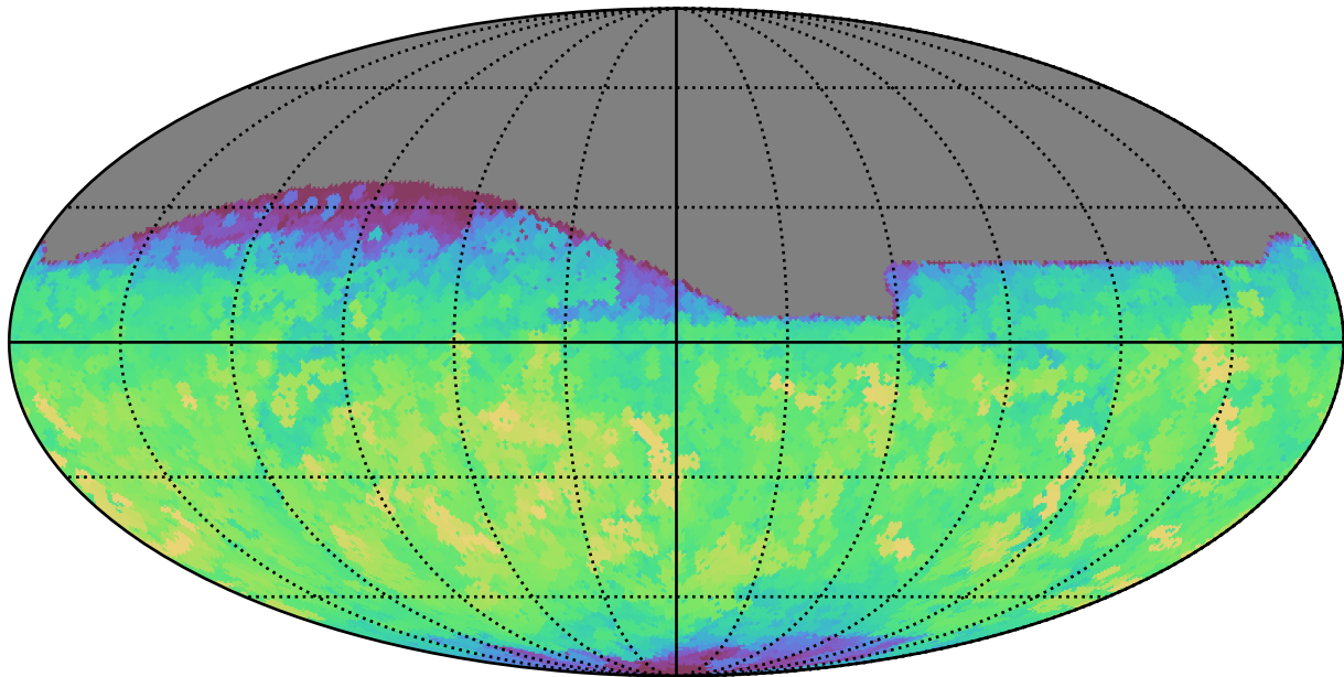
weather_cloudso8v3.4_10yrs All sky r band: Max saturation_mag
