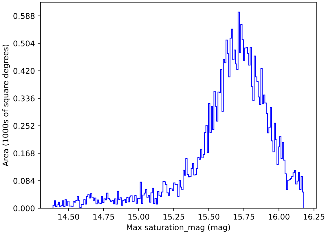
weather_cloudso8v3.4_10yrs All sky r band: Max saturation_mag
