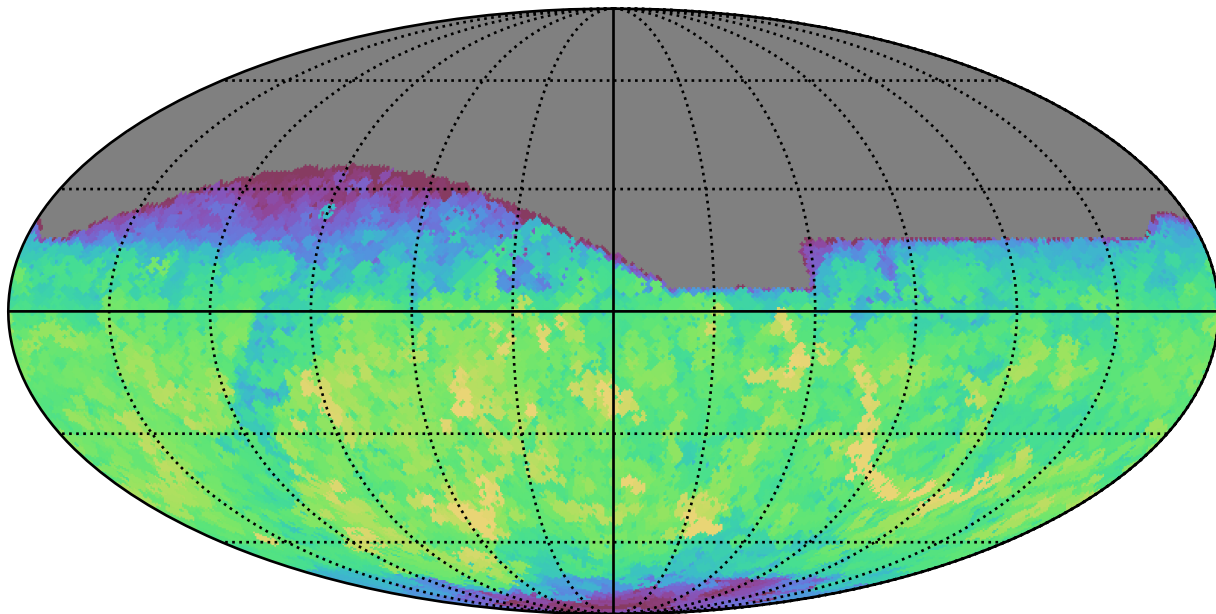
weather_cloudso8v3.4_10yrs All sky i band: Max saturation_mag
