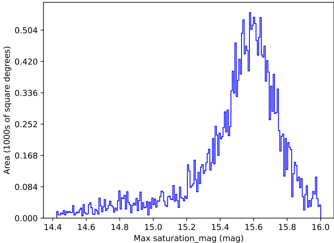
weather_cloudso8v3.4_10yrs All sky i band: Max saturation_mag
