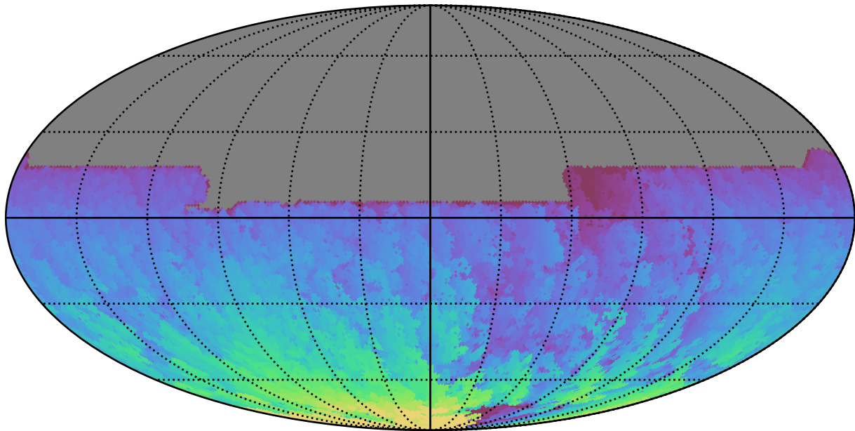
weather_cloudso8v3.4_10yrs All sky y band: Max HA
