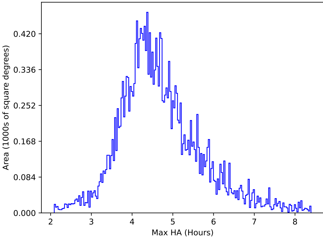
weather_cloudso8v3.4_10yrs All sky y band: Max HA
