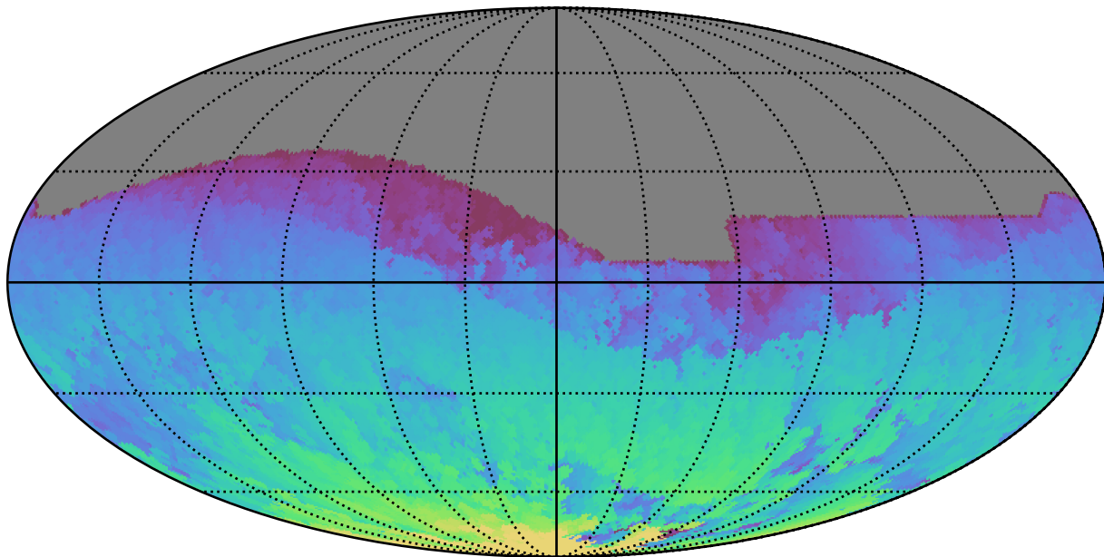
weather_cloudso8v3.4_10yrs All sky i band: Max HA
