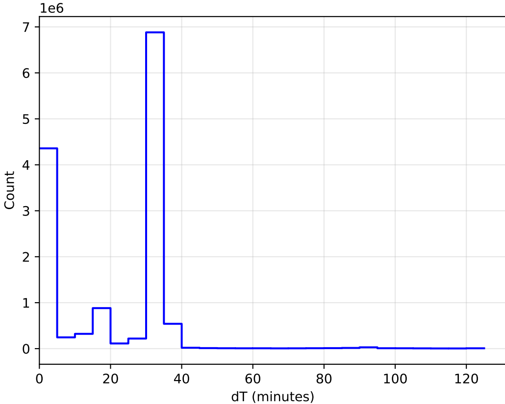
weather_cloudso8v3.4_10yrs All sky: DeltaT Histogram
