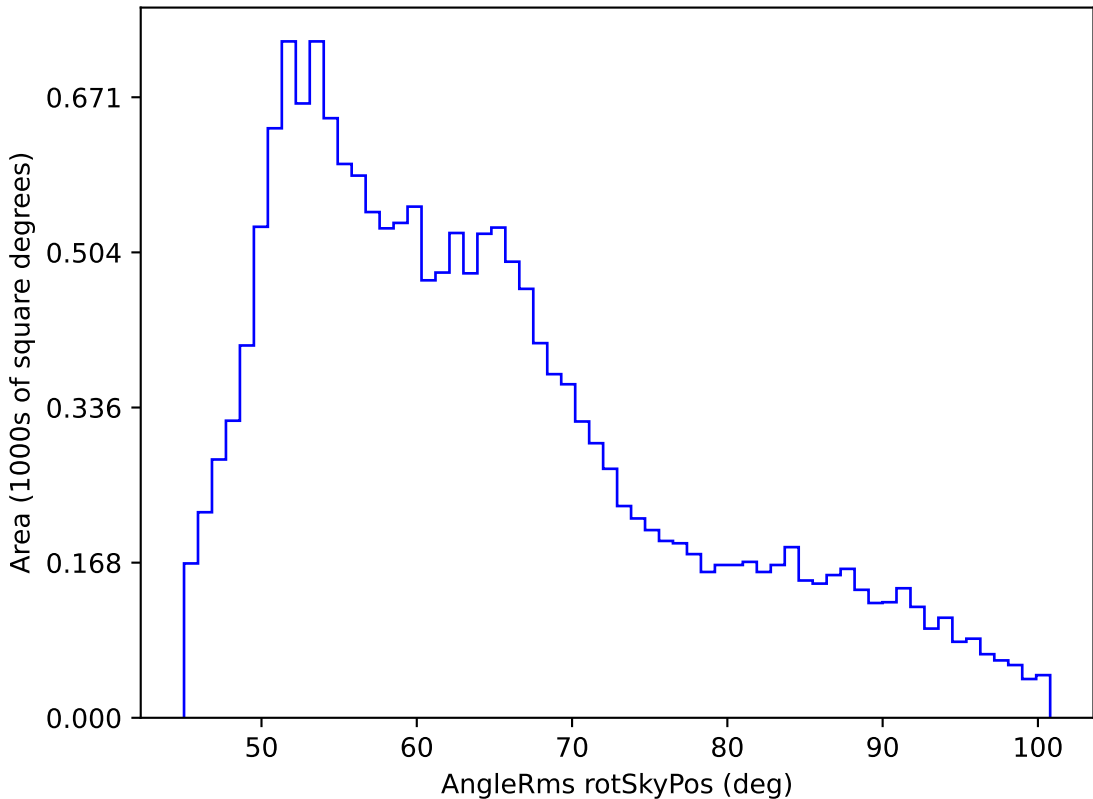
weather_cloudso8v3.4_10yrs WFD y band: AngleRms rotSkyPos
