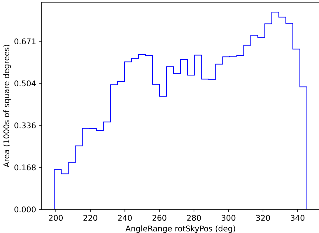
weather_cloudso8v3.4_10yrs WFD z band: AngleRange rotSkyPos
