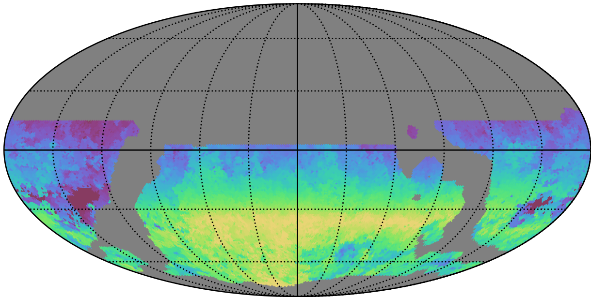
weather_cloudso8v3.4_10yrs WFD y band: AngleRange rotSkyPos
