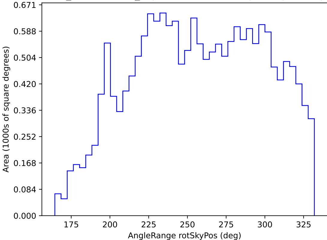
weather_cloudso8v3.4_10yrs WFD u band: AngleRange rotSkyPos
