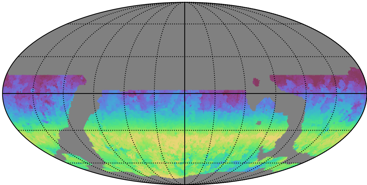
weather_cloudso8v3.4_10yrs WFD r band: AngleRange rotSkyPos
