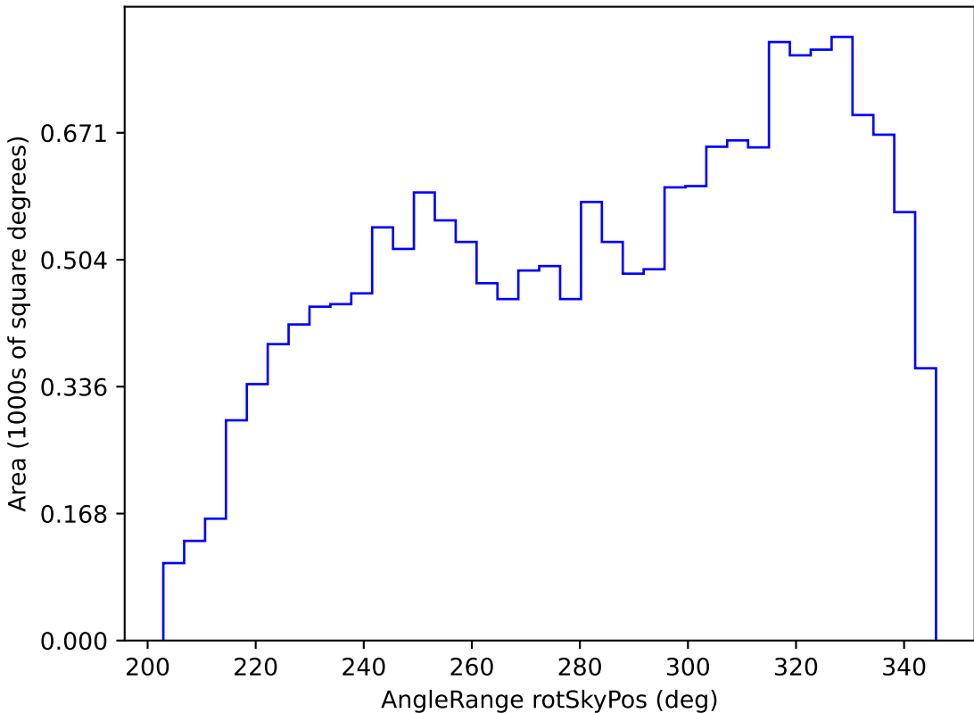
weather_cloudso8v3.4_10yrs WFD i band: AngleRange rotSkyPos
