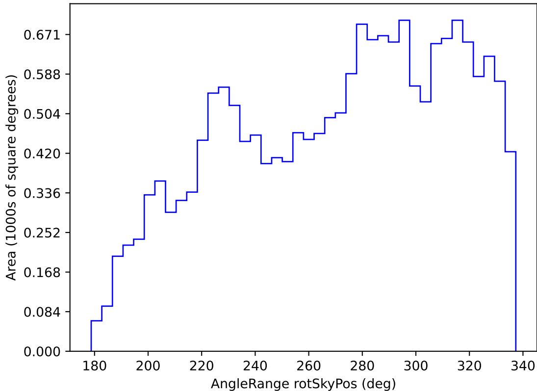
weather_cloudso8v3.4_10yrs WFD g band: AngleRange rotSkyPos
