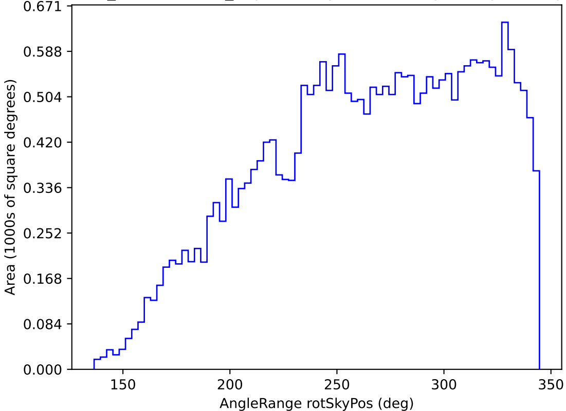
weather_cloudso8v3.4_10yrs All sky z band: AngleRange rotSkyPos
