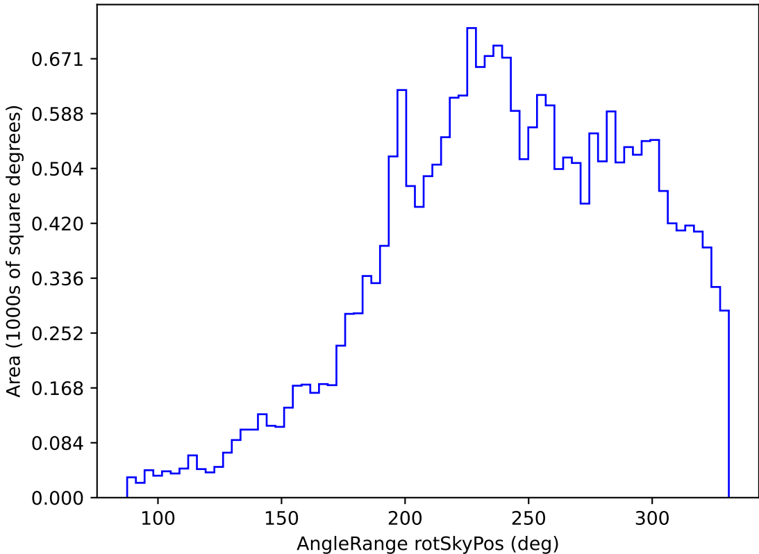
weather_cloudso8v3.4_10yrs All sky u band: AngleRange rotSkyPos
