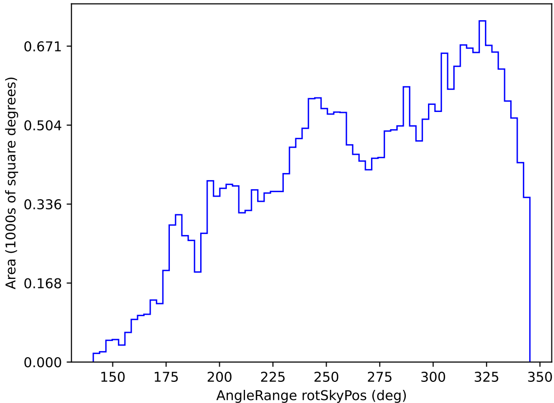
weather_cloudso8v3.4_10yrs All sky r band: AngleRange rotSkyPos
