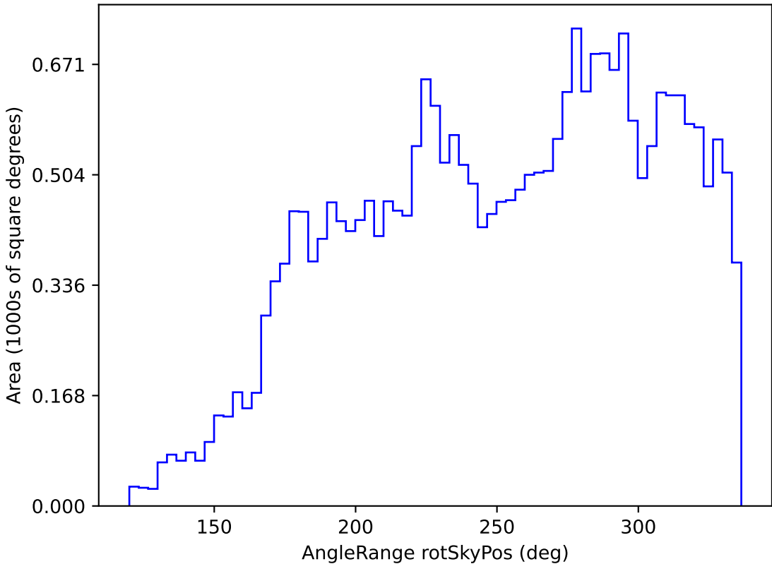
weather_cloudso8v3.4_10yrs All sky g band: AngleRange rotSkyPos
