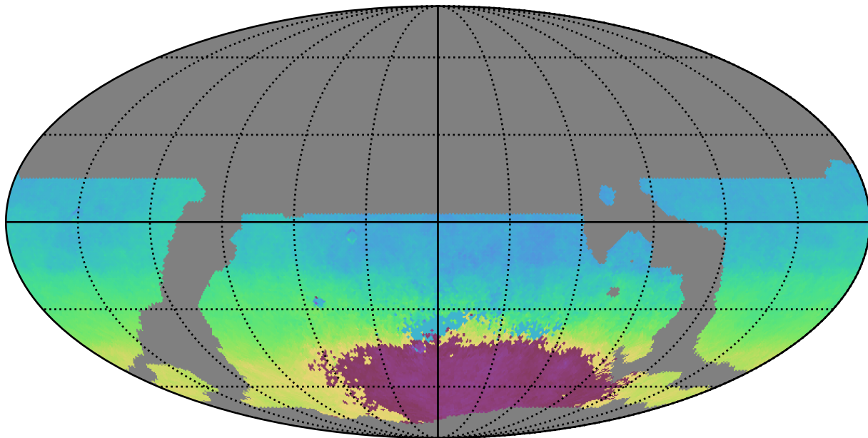
weather_cloudso8v3.4_10yrs WFD y band: AngleMean rotSkyPos
