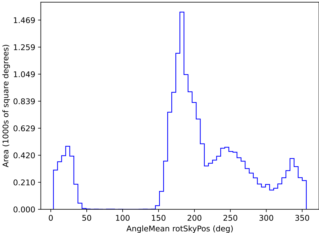
weather_cloudso8v3.4_10yrs WFD y band: AngleMean rotSkyPos
