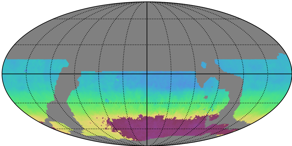
weather_cloudso8v3.4_10yrs WFD i band: AngleMean rotSkyPos
