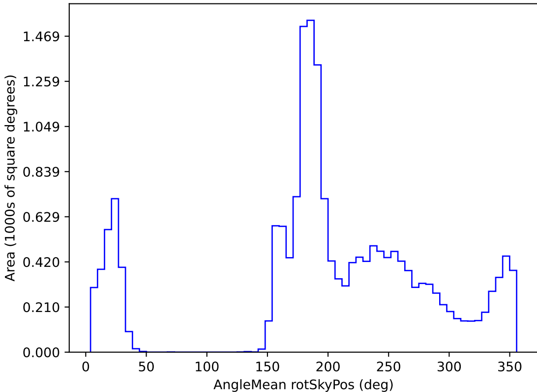
weather_cloudso8v3.4_10yrs WFD i band: AngleMean rotSkyPos
