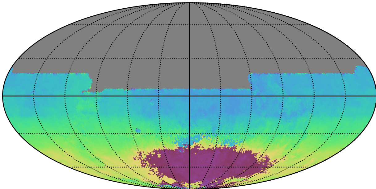
weather_cloudso8v3.4_10yrs All sky y band: AngleMean rotSkyPos
