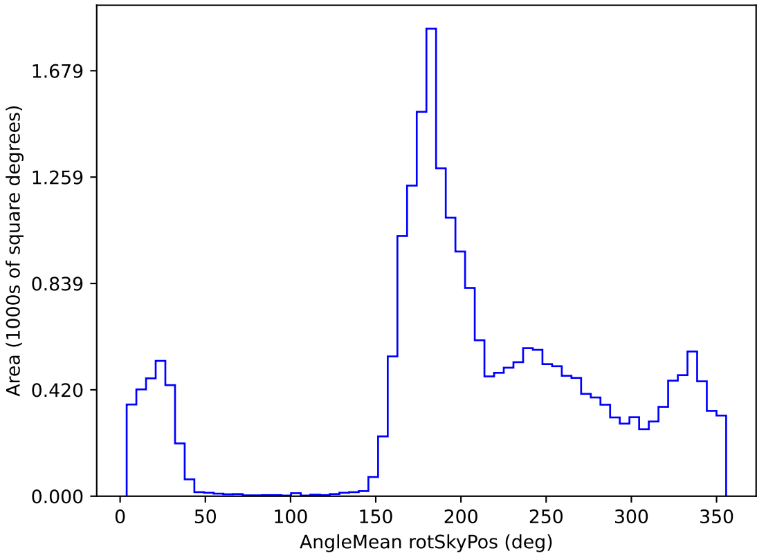
weather_cloudso8v3.4_10yrs All sky y band: AngleMean rotSkyPos
