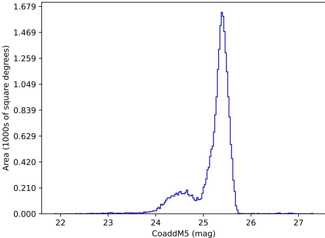
weather_cloudso8v3.4_10yrs u: CoaddM5
