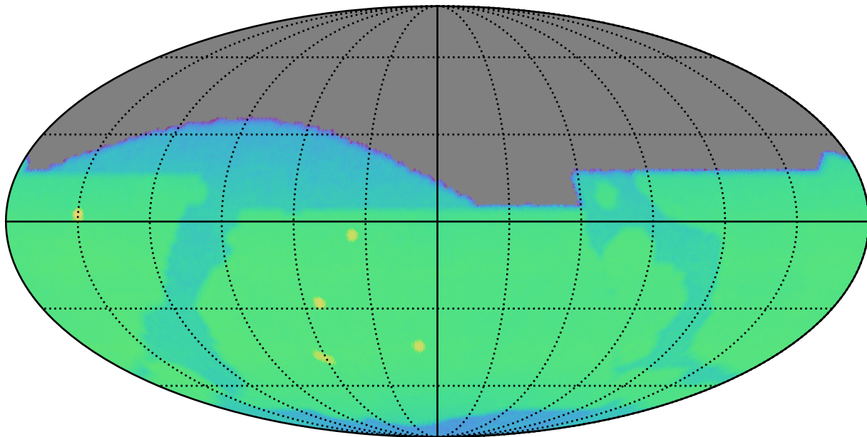
weather_cloudso8v3.4_10yrs i: CoaddM5
