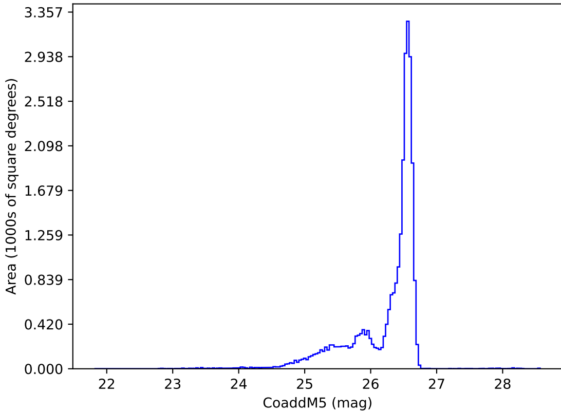
weather_cloudso8v3.4_10yrs i: CoaddM5
