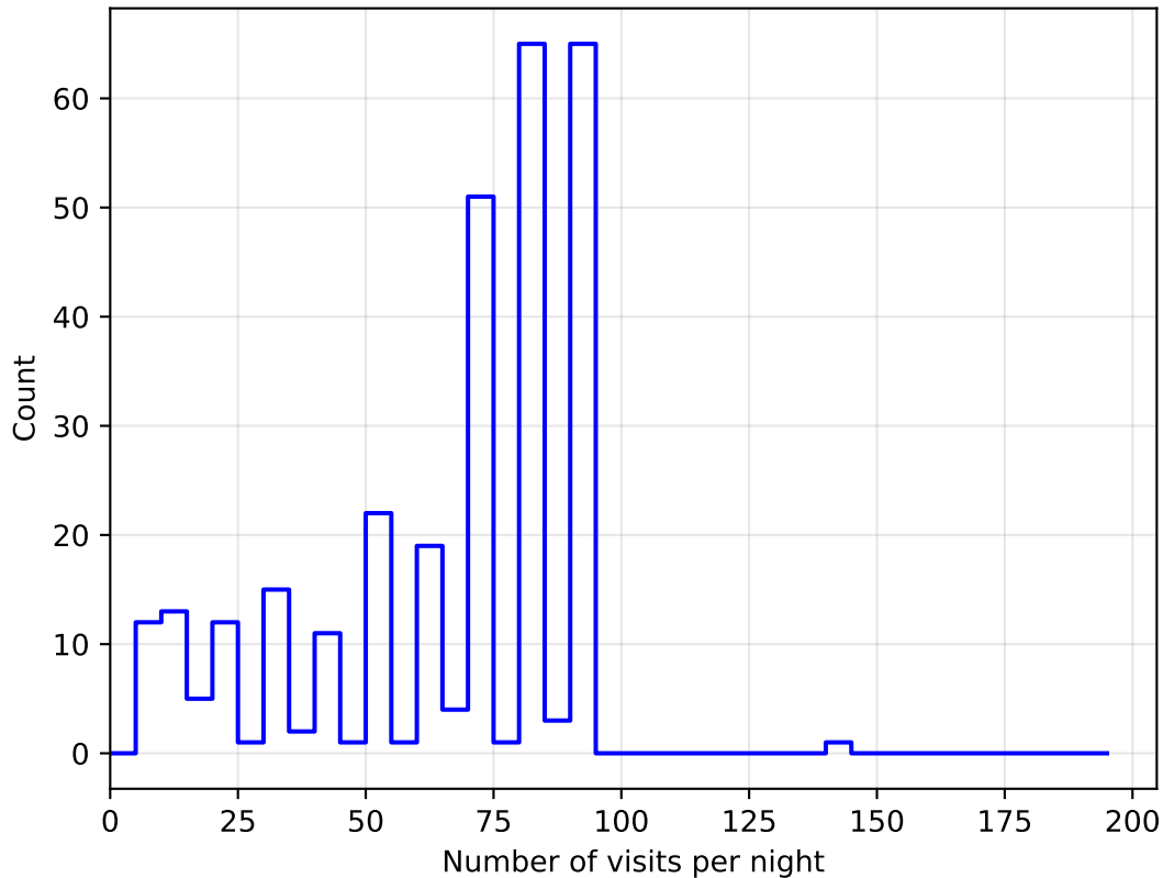
weather_cloudso8v3.4_10yrs all bands: DD:ELAISS1 NVisitsPerNight
