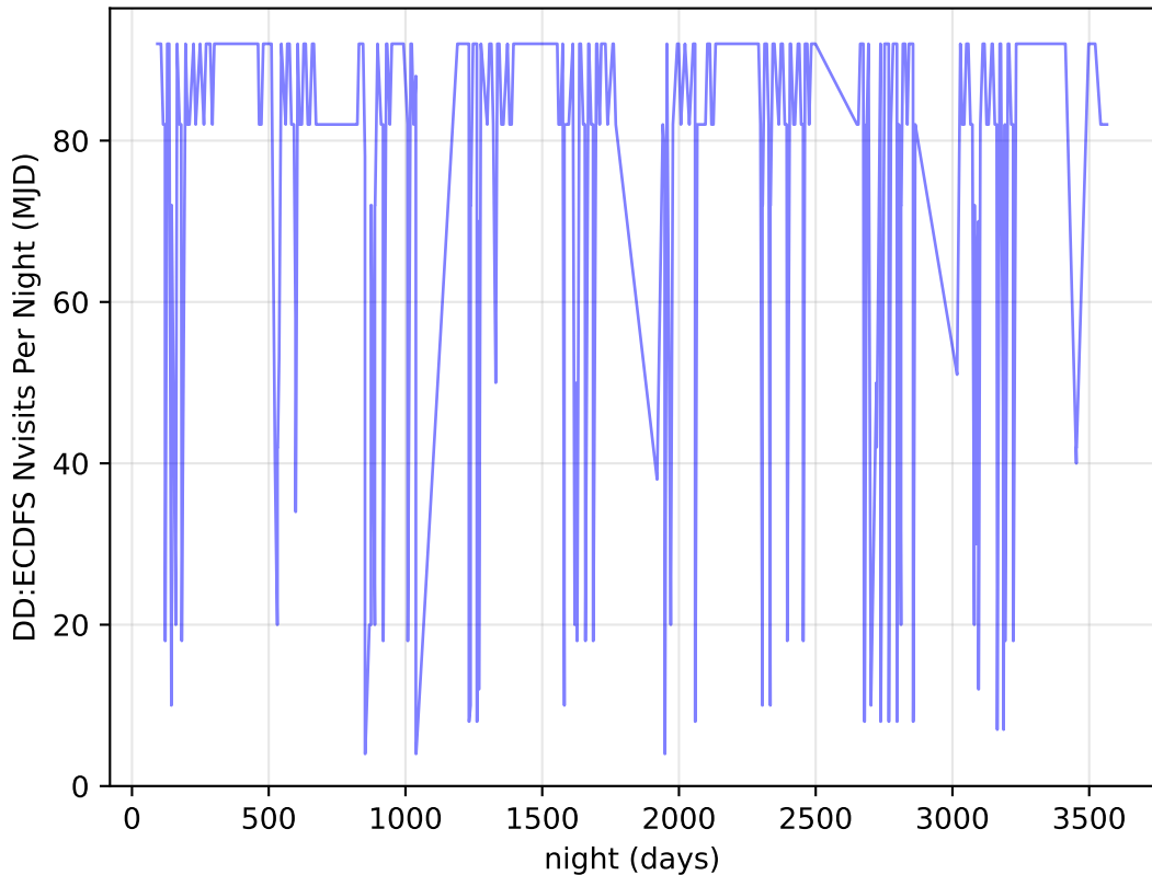
weather_cloudso8v3.4_10yrs all bands: DD:ECDFS Nvisits Per Night
