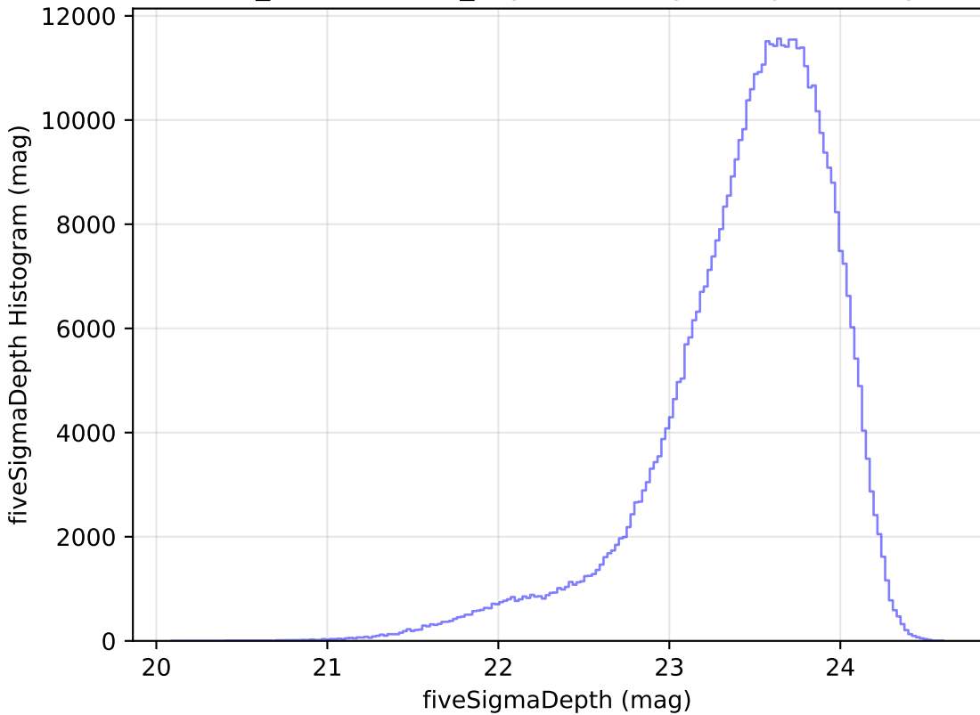
weather_cloudso6v3.4_10yrs i: fiveSigmaDepth Histogram
