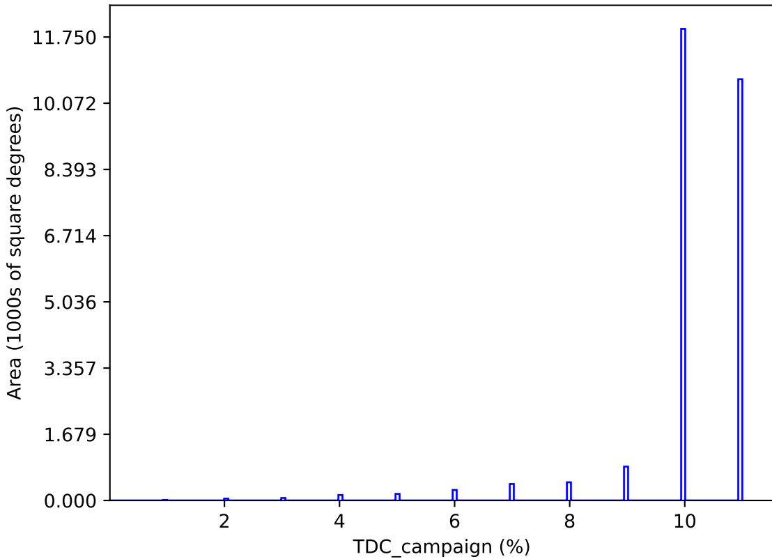
weather_cloudso6v3.4_10yrs : TDC_campaign
